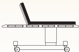
Inclinazione schienale
